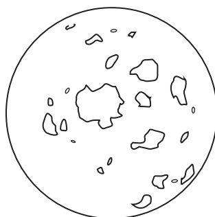
Mars
